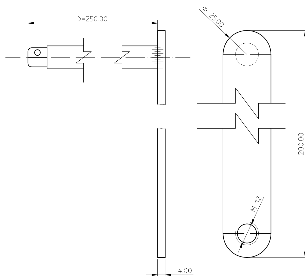
MARCA 8- CUERPO MANERAL ESCALA 1:1
