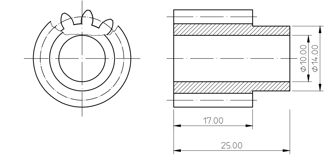
MARCA 1- ENGRANAJE ESCALA 2:1
