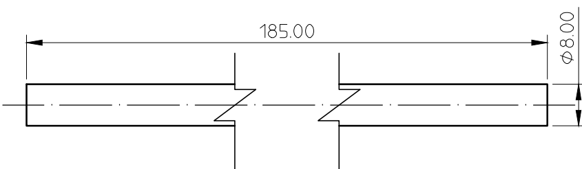
MARCA 3- TOPE ESCALA 1:1
