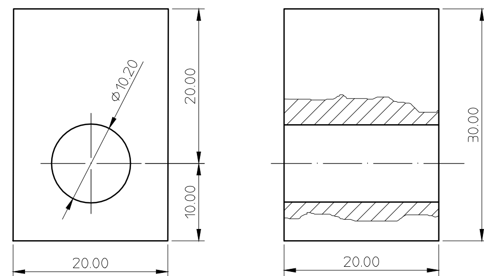
MARCA 5- SOPOTE APOYO ESCALA 2:1
