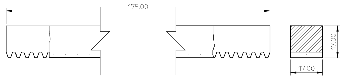
MARCA 2- CREMALLERA ESCALA 2:1
