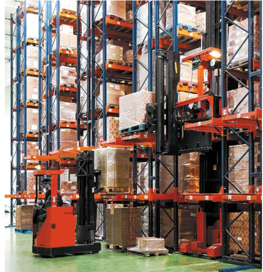
Almacén dedicado a maquinaria y herramientas para la construcción. Fuente: Mecalux.
