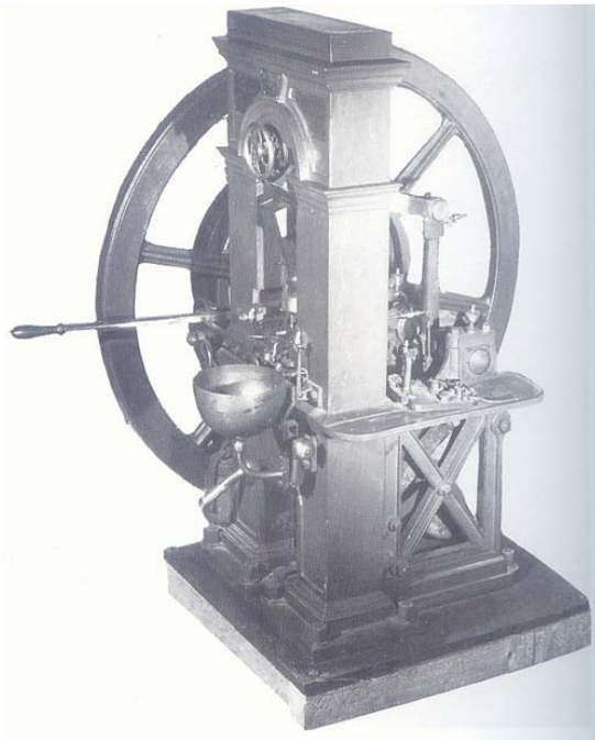
Ilustración 35 – Prensa Thonnelier
